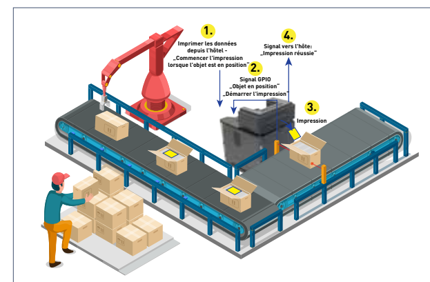
Synchronisation du système avec GPIO
